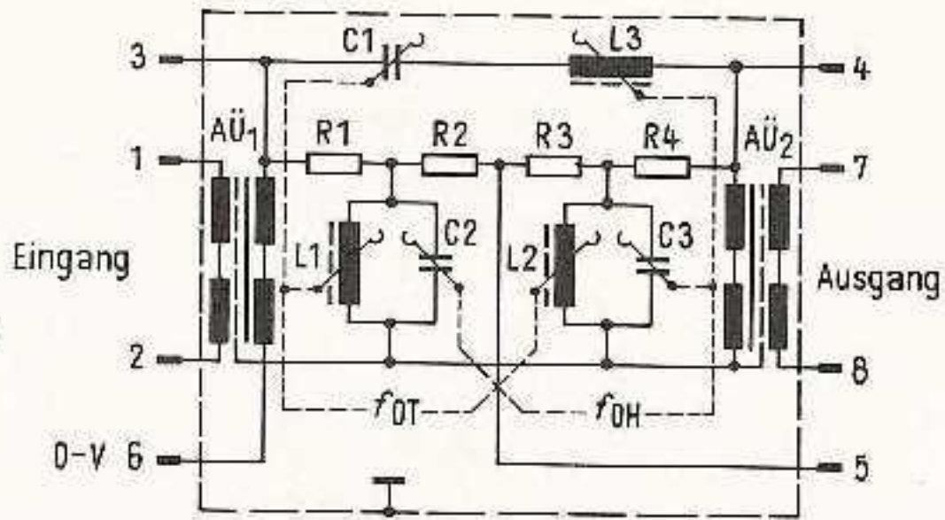
Bild 144. Hörspiel- verzerrer HV 55 (Eckmiller)
