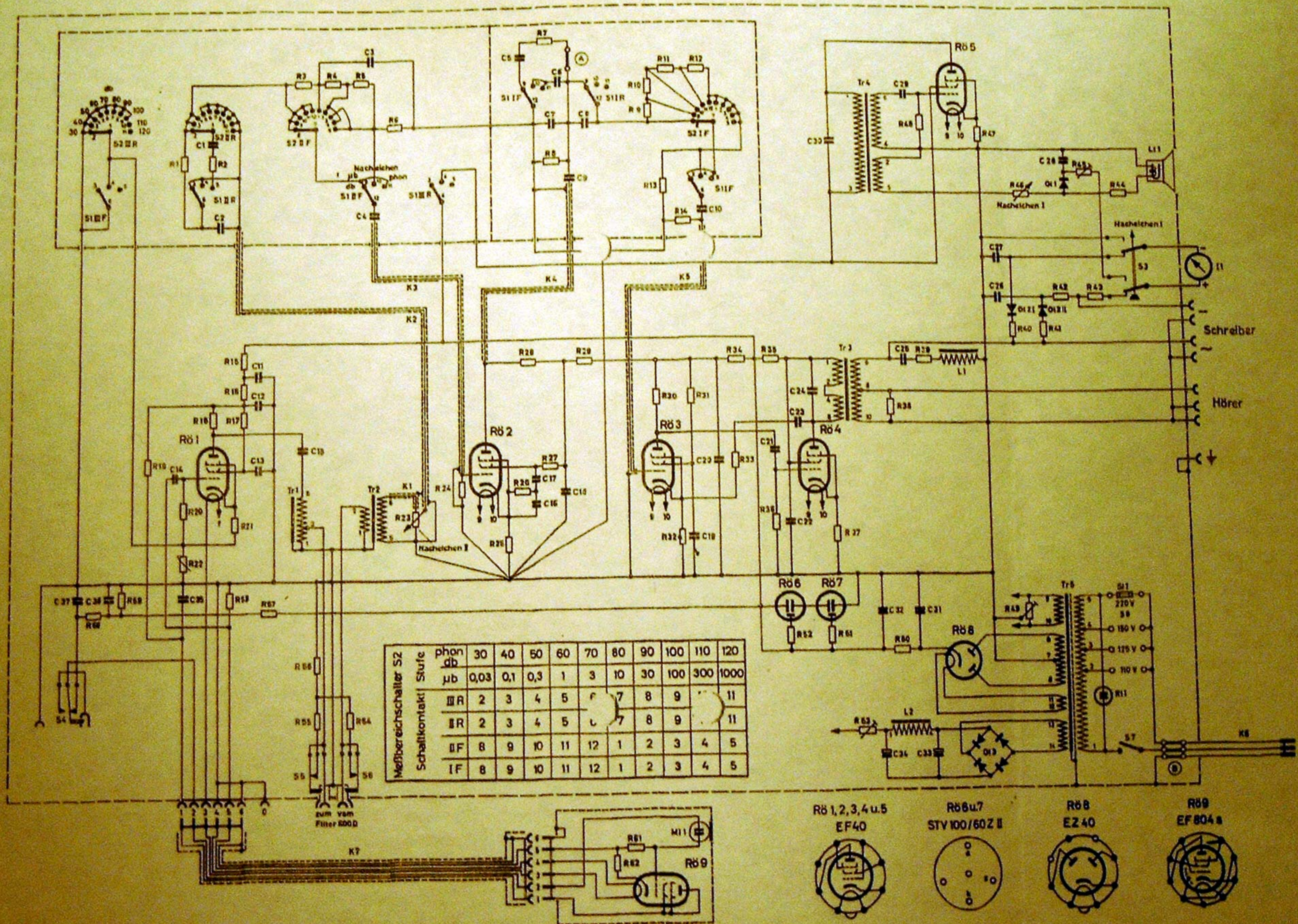
Abb. 2. Stromlauf des Schallpegelmessers Type EZGN BN 4502
